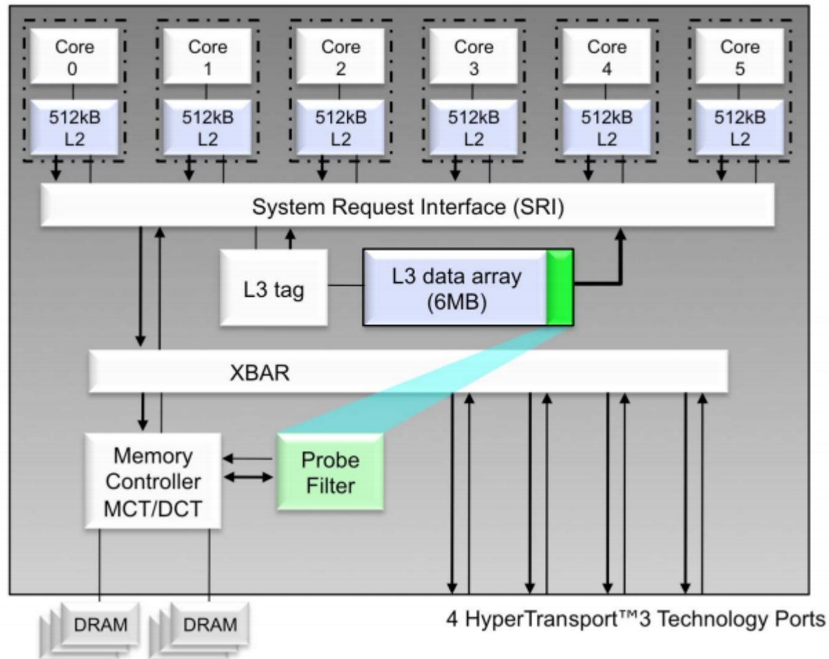
“Magny-Cours” Die (Node)
