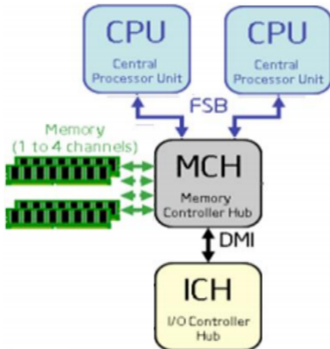
Intel's FSB based UMA Arch.
