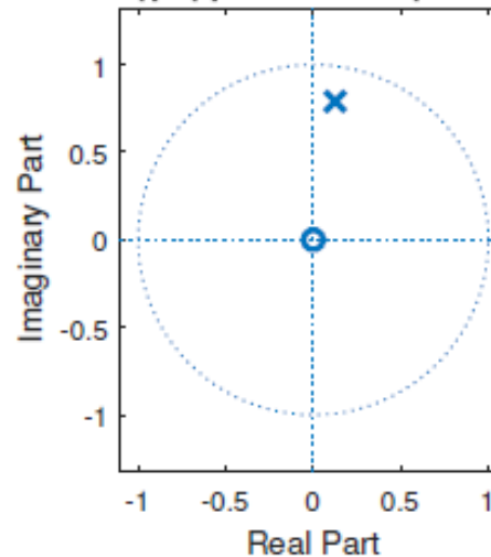
Διάγραμμα Πόλων-Μηδενικών
