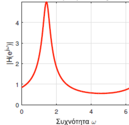
Απόκριση Πλάτους
