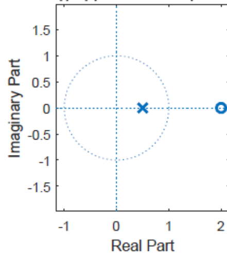
Διάγραμμα Πόλων-Μηδενικών
