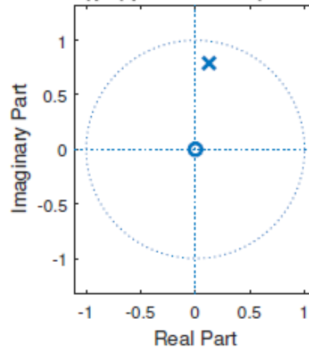
Διάγραμμα Πόλων-Μηδενικών
