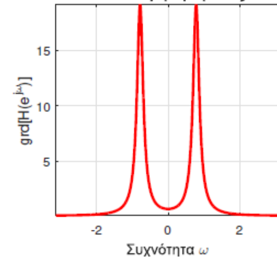
Καθυστέρηση Ομάδας
