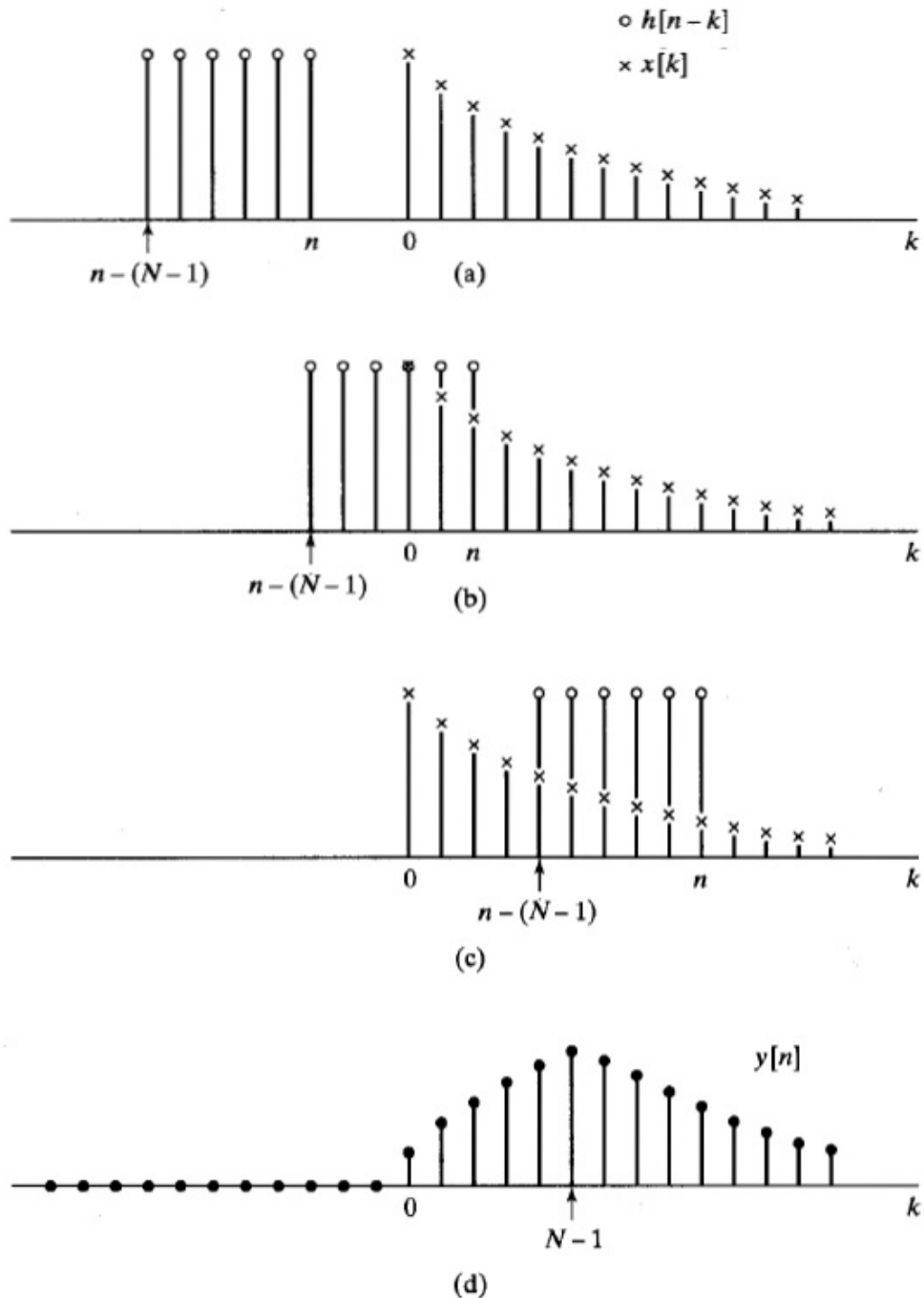
Σχήμα 12.3: Σήματα x[n] και h[n - k] για τον υπολογισμό συνέλιξης. Στα (a - c) βλέπετε τα σήματα x[n] και h[n - k] ως συνάρτηση του k για διάφορες τιμές του n . Στο (d) βλέπετε το σήμα εξόδου ως συνάρτηση του n .
