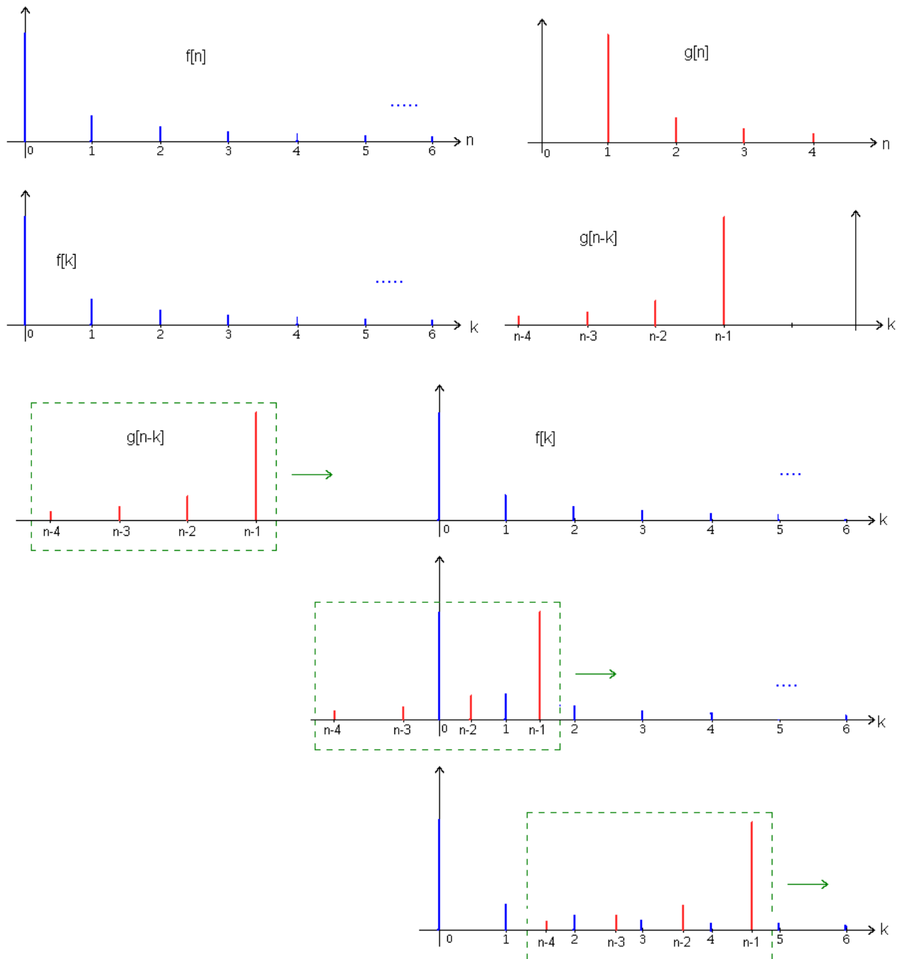
Σχήμα 12.2: Διαδικασία συνέλιξης διακριτού χρόνου.
