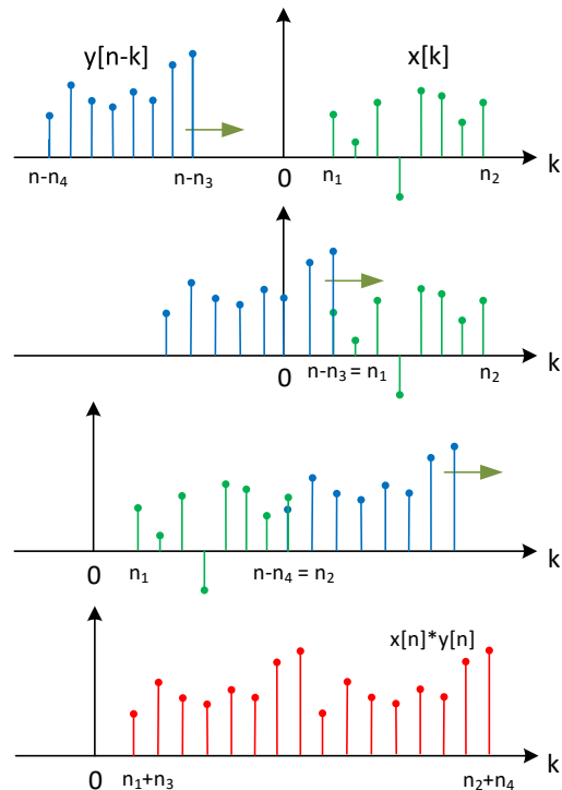
Σχήμα 12.1: Γραφική απόδειξη της ιδιότητας του εύρους.
