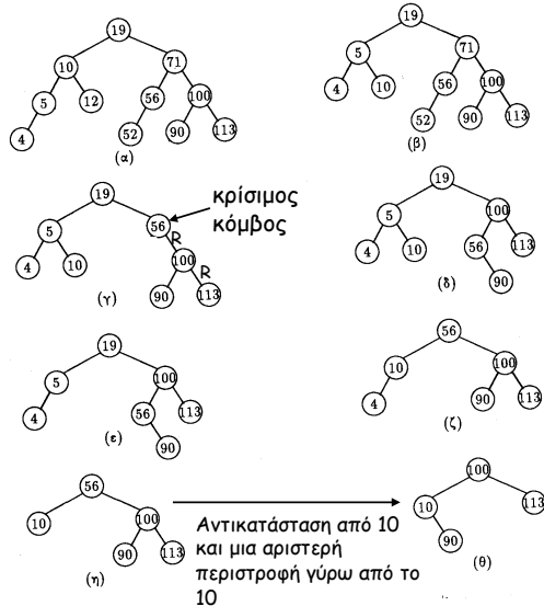
Σχήμα 5.3: Ι. Μανωλόπουλος, Δομές Δεδομένων, Μια προσέγγιση με την Pascal, Εκδόσεις Art of Text.
