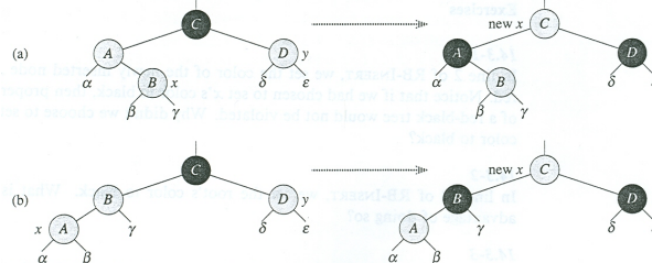
Σχήμα 13.5: Cormen, Leiserson, Rivest & Stein, Εισαγωγή στους Αλγορίθμους, Πανεπιστημιακές Εκδόσεις Κρήτης, 2006
