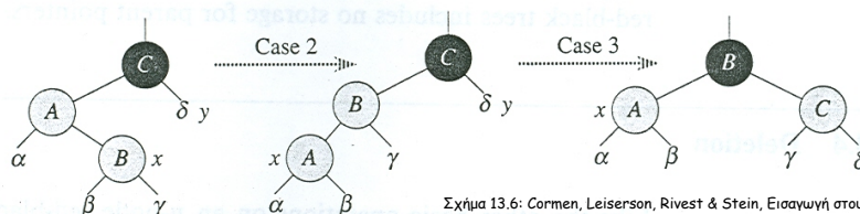
Σχήμα 13.6: Cormen, Leiserson, Rivest & Stein, Εισαγωγή στους Αλγορίθμους, Πανεπιστημιακές Εκδόσεις Κρήτης, 2006
