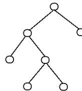
Γεμάτο Δυαδικό Δένδρο
