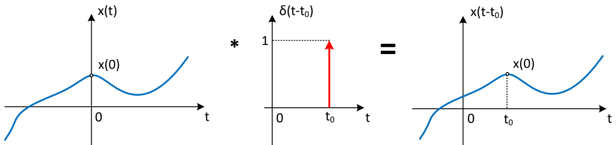
Σχήμα 3.17: Συνέλιξη σήματος με συνάρτησης Δέλτα.
