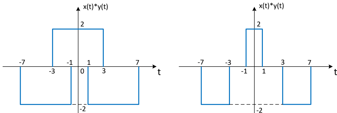
Σχήμα 3.20: Παράδειγμα συνέλιξης σήματος με Συνάρτηση Δέλτα: συνέλιξη σημάτων.
