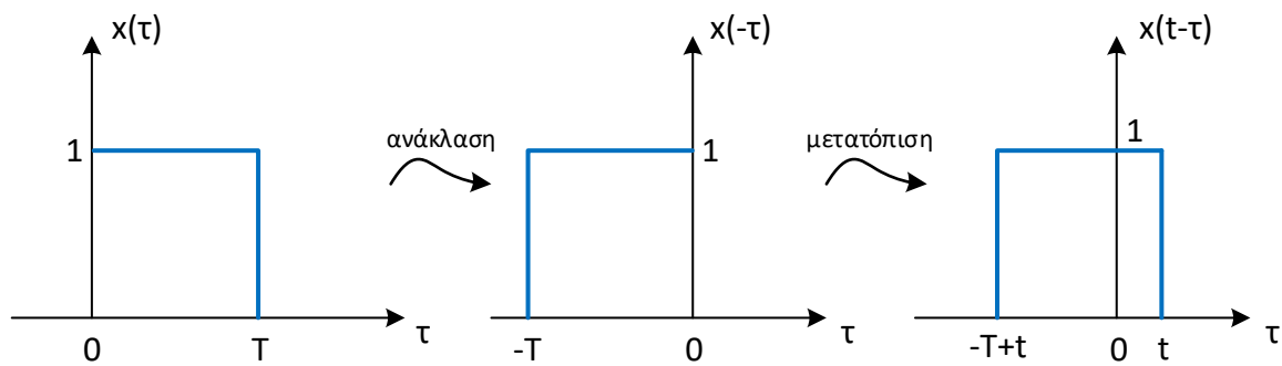
Σχήμα 3.10: Μετατόπιση και ανάκλαση σήματος x(t) .
