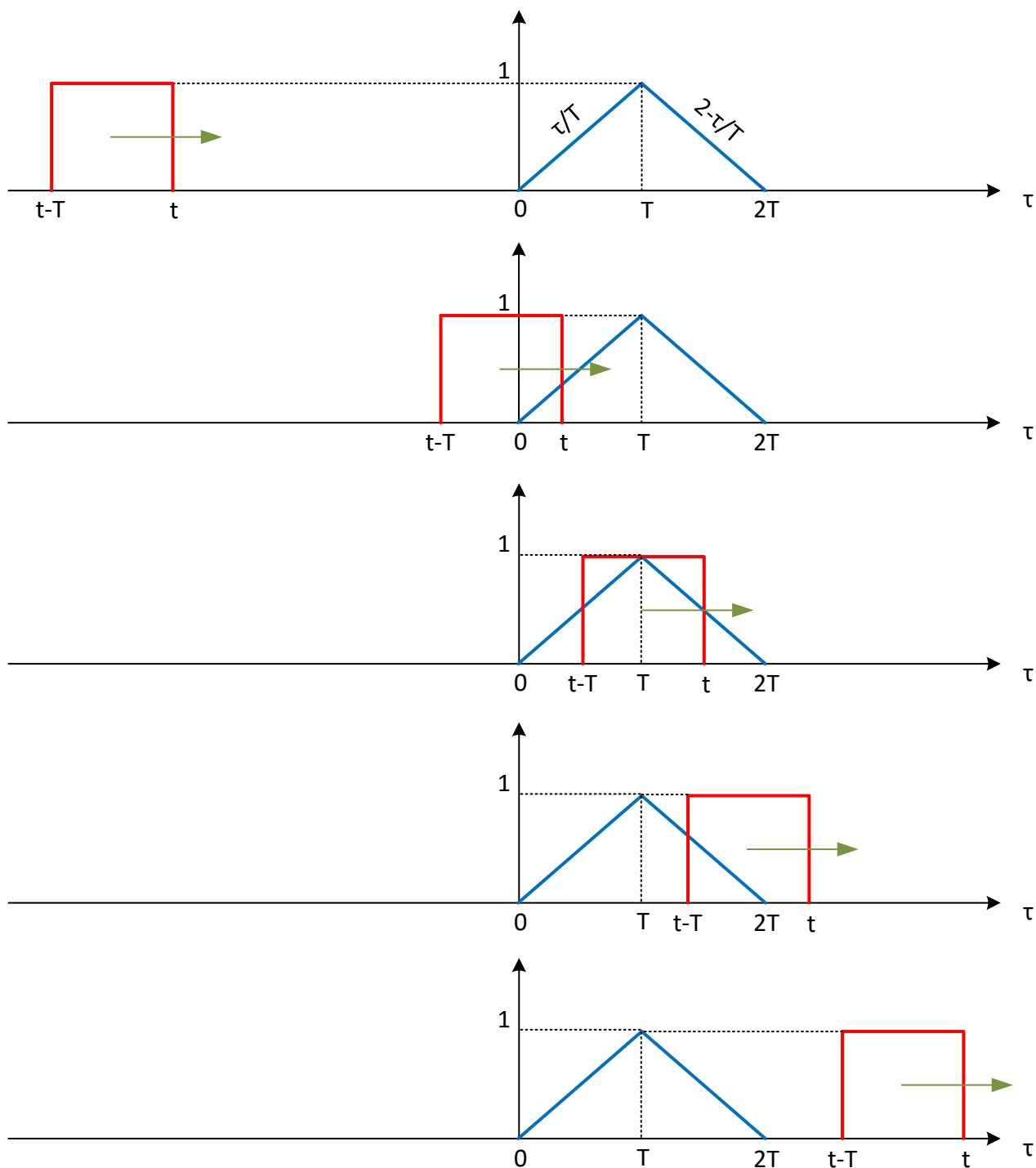
Σχήμα 3.11: Περιπτώσεις Συνέλιξης Παραδείγματος 3.8.
