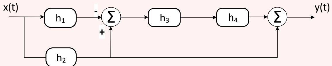
Σχήμα 3.26: Διάταξη Συστημάτων Παραδείγματος 3.17.
