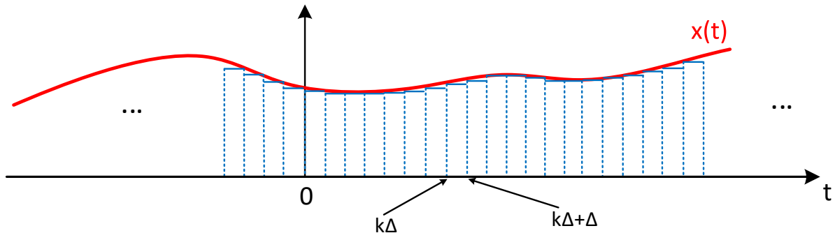
Σχήμα 3.6: Προσέγγιση σήματος x(t) από σήματα \Delta x(k\Delta)\delta_\Delta(t - k\Delta) .
