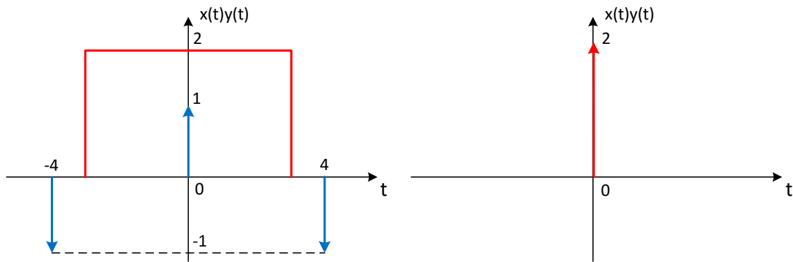
Σχήμα 3.19: Παράδειγμα συνέλιξης σήματος με Συνάρτηση Δέλτα: γινόμενο σημάτων.
