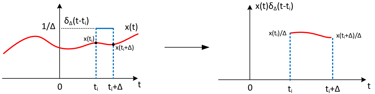
Σχήμα 3.5: Σήμα x(t)\delta_\Delta(t - t_i) .
