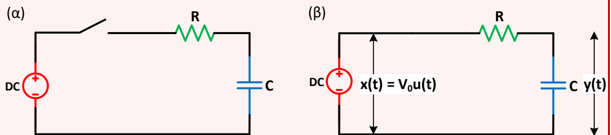
Σχήμα 3.23: Κύκλωμα RC Παραδείγματος 3.16.
