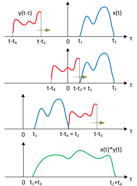
Σχήμα 3.7: Γραφική απόδειξη της ιδιότητας του εύρους.
