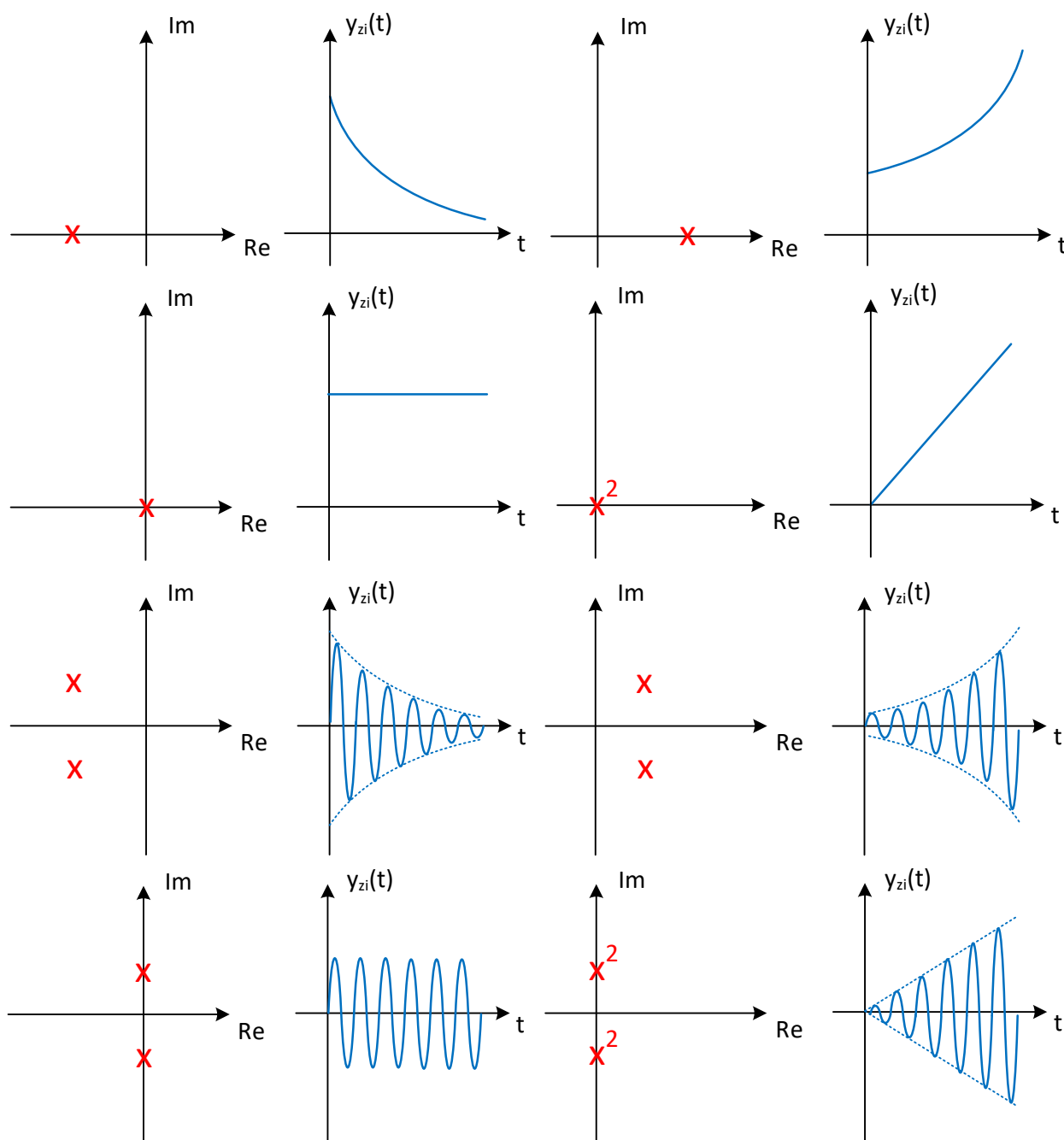
Σχήμα 3.22: Θέσεις χαρακτηριστικών ριζών και μορφή απόκρισης μηδενικής εισόδου.
