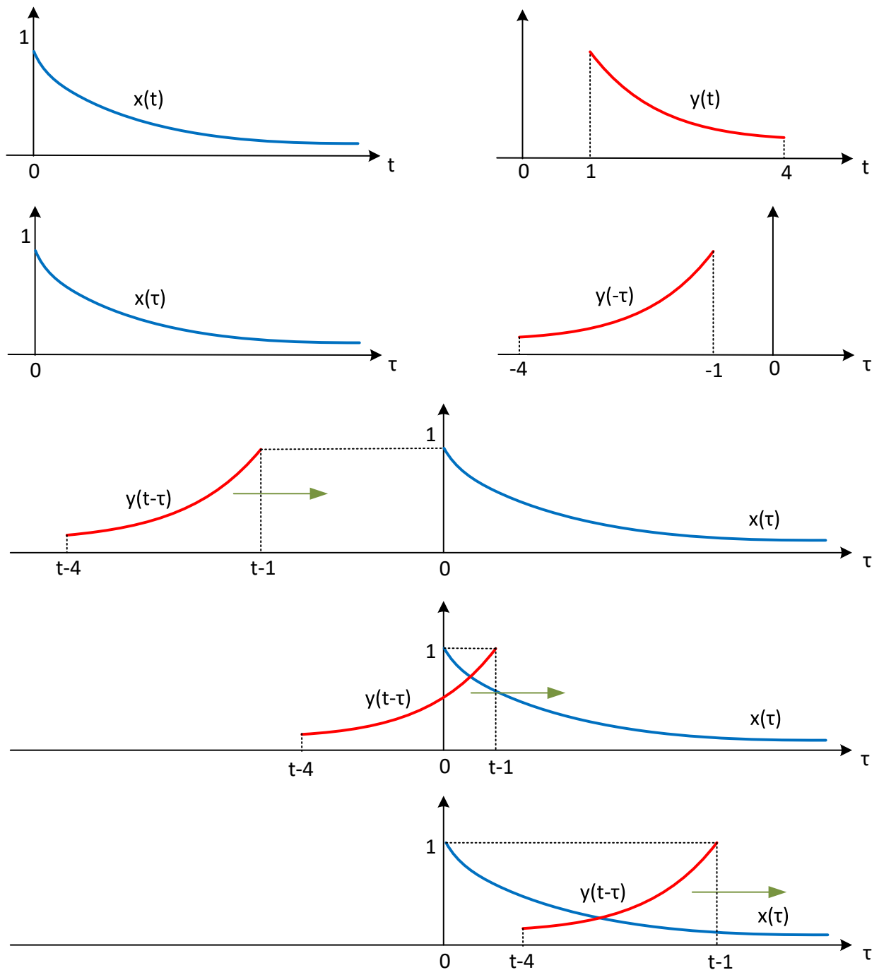
Σχήμα 3.8: Γραφική απεικόνιση της συνέλιξης.
