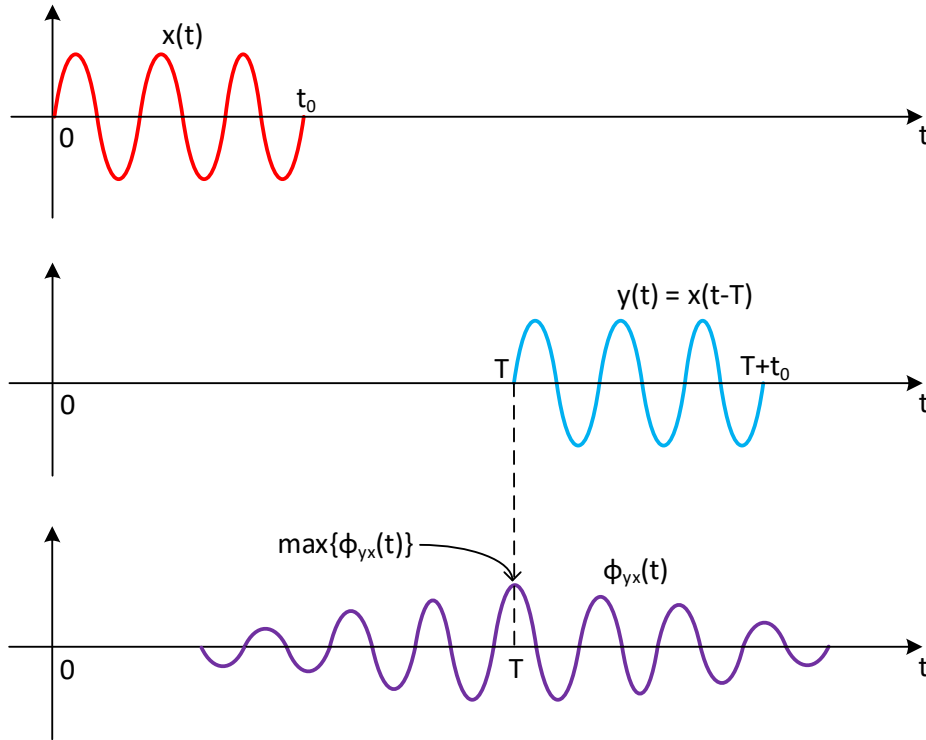
Σχήμα 5.1: Εκπεμπόμενο και ληφθέν σήμα σε ένα radar.
