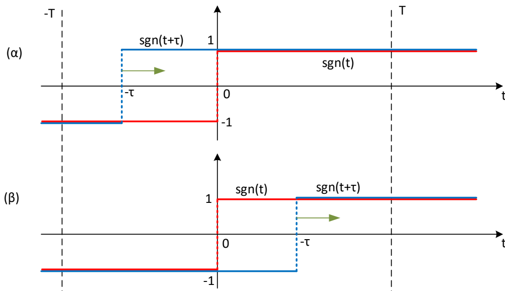
Σχήμα 5.4: Περιπτώσεις στον υπολογισμό της αυτοσυσχέτισης του x(t) = \text{sgn}(t) .
