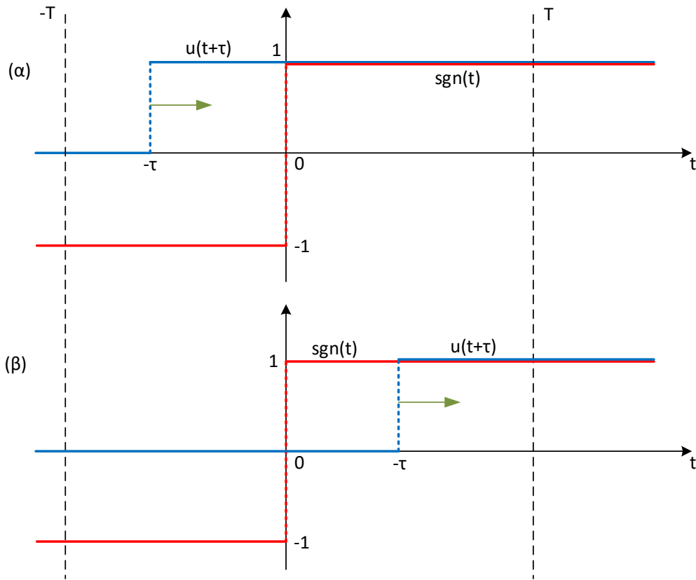
Σχήμα 5.6: Περιπτώσεις στον υπολογισμό της ετεροσυσχέτισης του x(t) = \text{sgn}(t) με το y(t) = u(t) .
