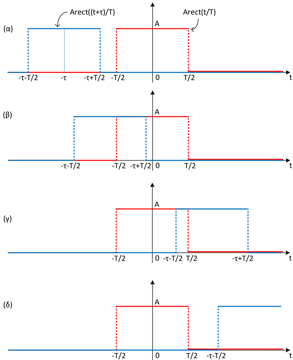
Σχήμα 5.5: Περιπτώσεις στον υπολογισμό της αυτοσυσχέτισης του x(t) = \text{Arect}\left(\frac{t}{T}\right) .
