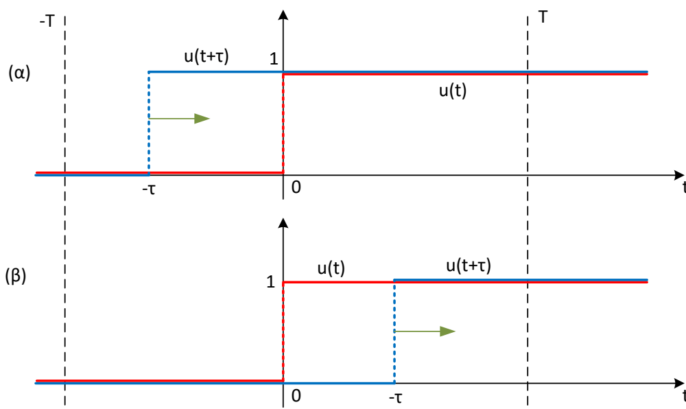
Σχήμα 5.3: Περιπτώσεις στον υπολογισμό της αυτοσυσχέτισης του x(t) = u(t) .
