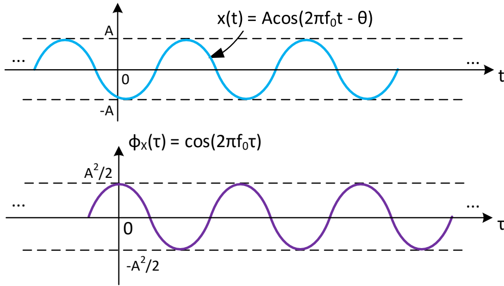
Σχήμα 5.2: Περιοδική αυτοσυσχέτιση ημιτόνου x(t) = A \cos(2\pi f_0 t - \theta) .
