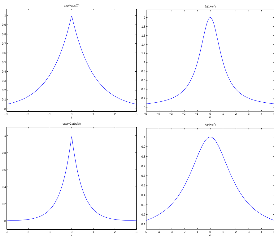
Σχήμα 4.2: Ο μετασχηματισμός Fourier του σήματος του Παραδείγματος 6.2.2 για δύο τιμές του \alpha .
