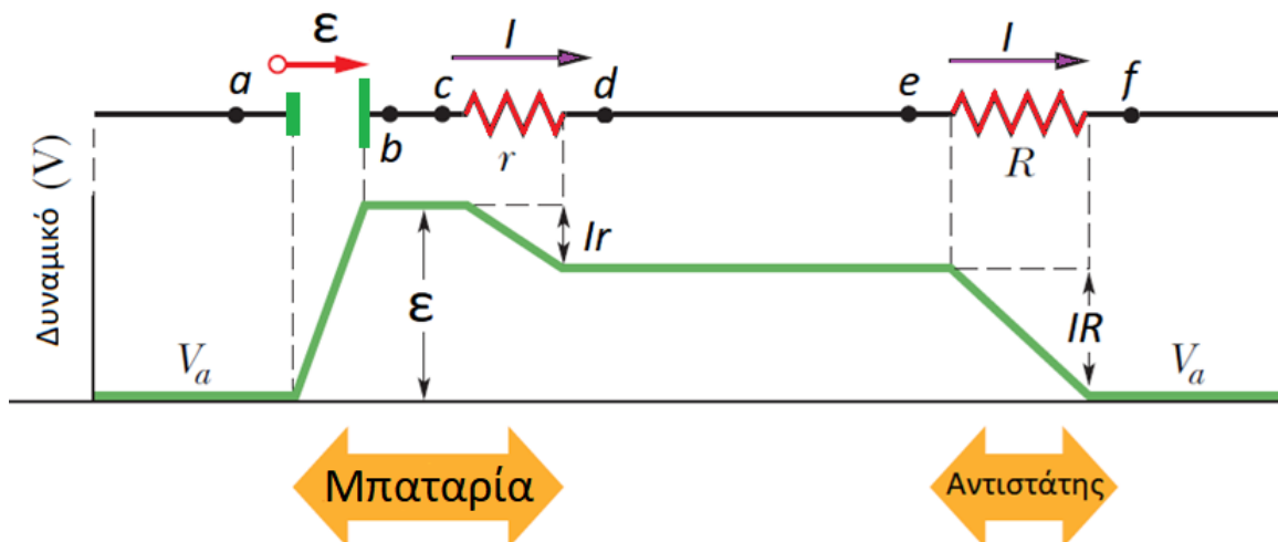
Σχήμα 4.73: Δυναμικά κατά μήκος κυκλώματος.
