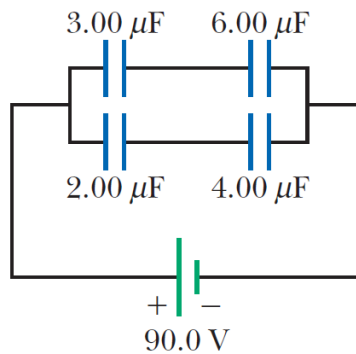
Σχήμα 4.61: Συνδυασμός Πυκνωτών.
