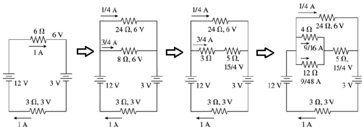
Σχήμα 4.130: Σχήμα Άσκησης 4.90- Σύνθεση του αρχικού κυκλώματος.
