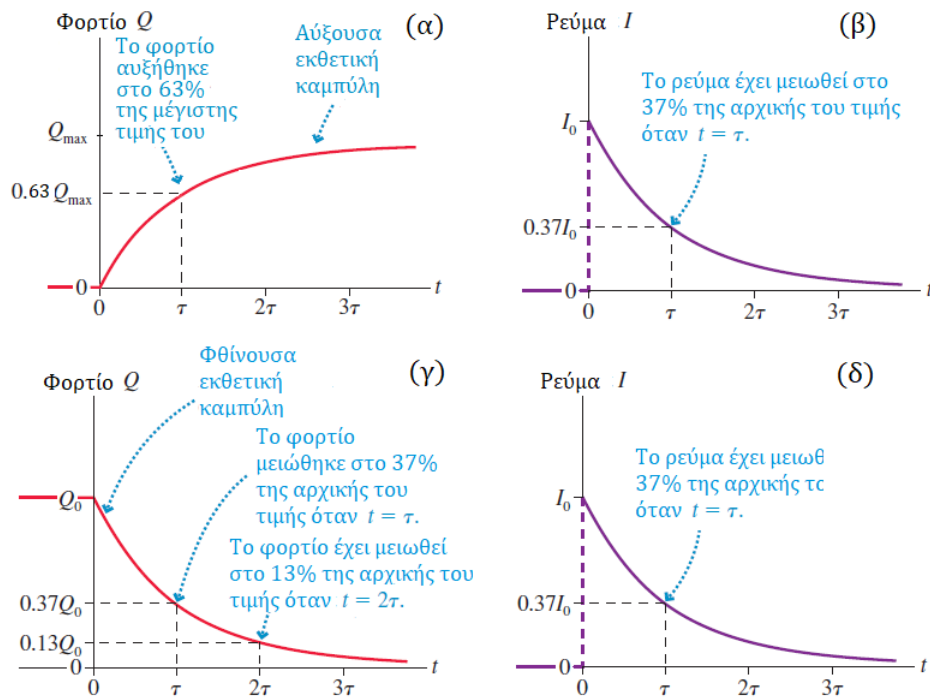
Σχήμα 4.85: Ρεύματα και φορτία σε κύκλωμα RC .
