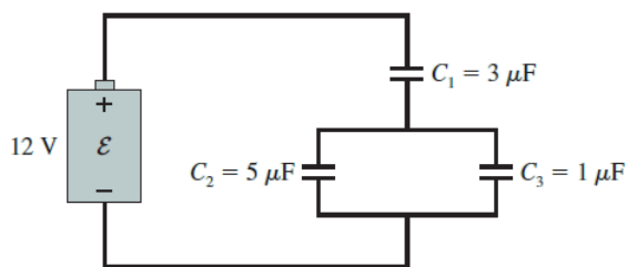
Σχήμα 4.59: Κύκλωμα πυκνωτών.
