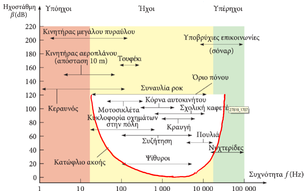
Σχήμα 3.32: Ηχοστάθμη συναρτήσει της συχνότητας.
