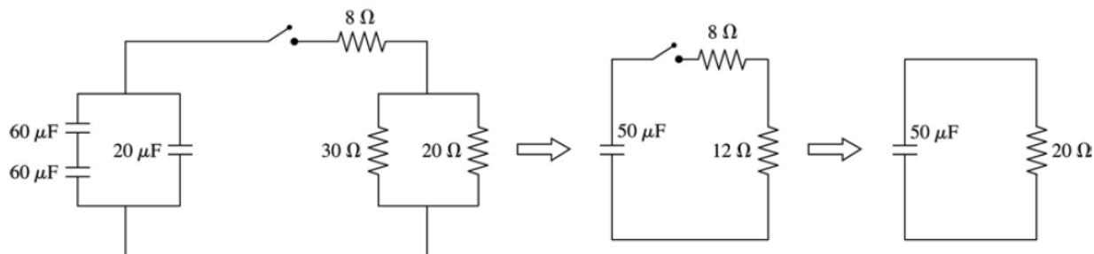
Σχήμα 4.140: Απλοποίηση κυκλώματος Άσκησης 4.98.
