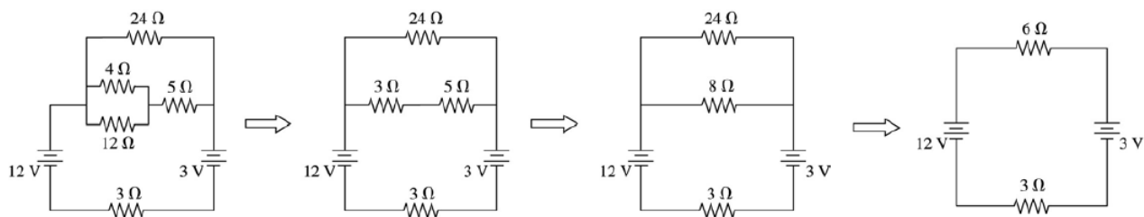
Σχήμα 4.129: Σχήμα Άσκησης 4.90- Απλοποίηση.
