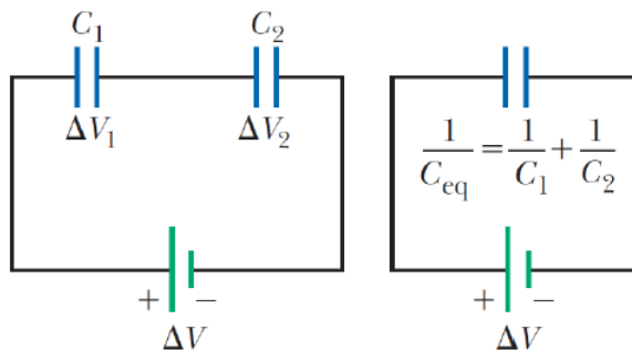
Σχήμα 4.58: Σειριακή Σύνδεση.
