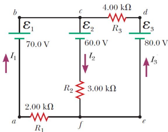
Σχήμα 4.79: Κύκλωμα και κανόνες Kirchhoff.
