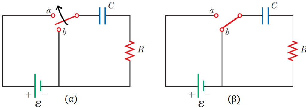
Σχήμα 4.84: Κύκλωμα RC.
