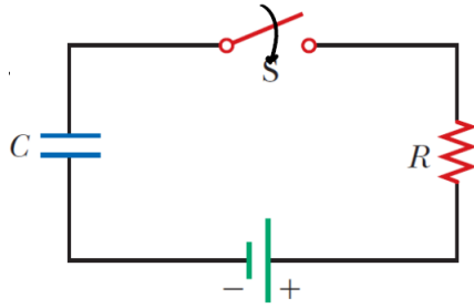
Σχήμα 4.86: Κύκλωμα RC.
