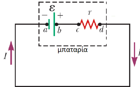
Σχήμα 4.71: Μοντέλο μπαταρίας σε κύκλωμα.
