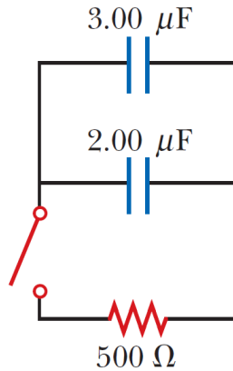
Σχήμα 4.88: Παράλληλοι πυκνωτές με αντιστάτη.
