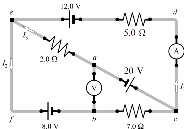
Σχήμα 4.136: Ηλεκτρικό κύκλωμα Άσκησης 4.94.
