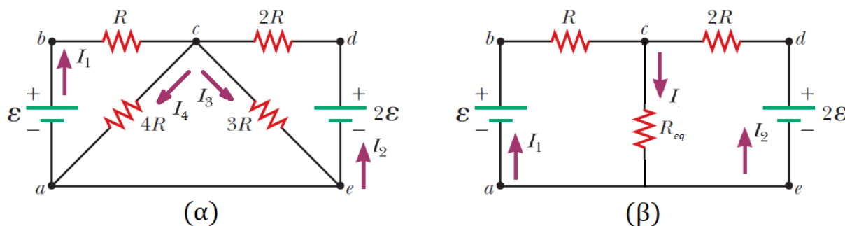
Σχήμα 4.77: Κύκλωμα και κανόνες Kirchhoff.
