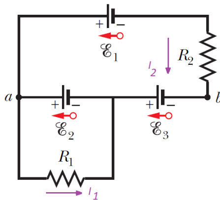
Σχήμα 4.81: Σχήμα Λύσης Άσκησης 4.44.
