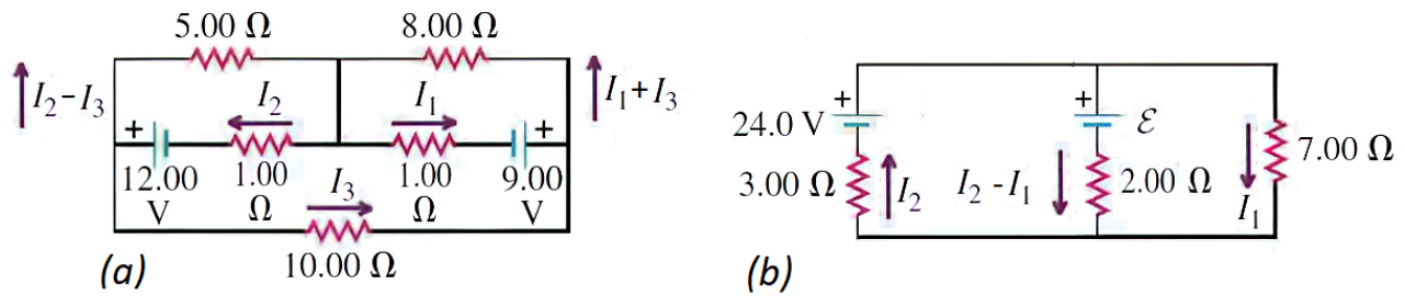
Σχήμα 4.134: Ανάλυση κυκλωμάτων Άσκησης 4.92.
