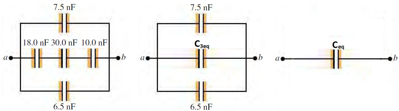
Σχήμα 4.127: Ανάλυση πυκνωτών Άσκησης 4.89.
