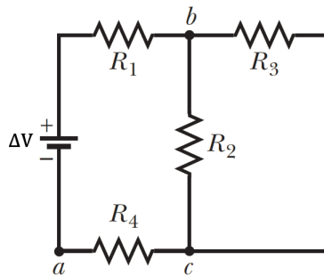
Σχήμα 4.66: Κύκλωμα αντιστατών.
