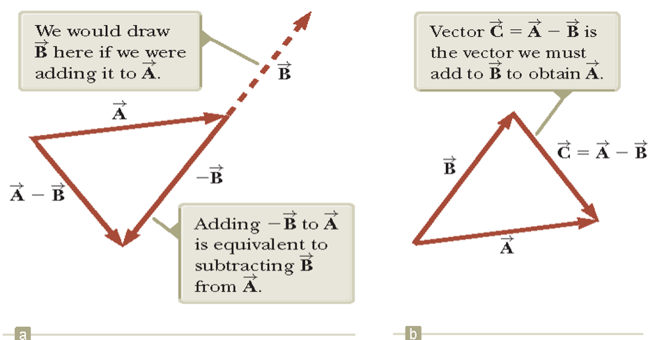
Σχήμα 1.5: Αφαίρεση διανυσμάτων.
