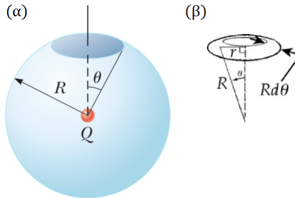
Σχήμα 4.101: Φορτίο σε σφαίρα.
