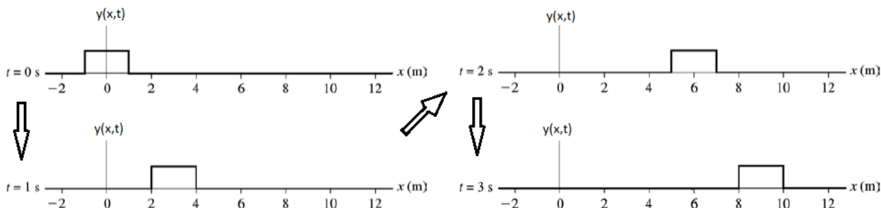
Σχήμα 3.23: Οδεύον κύμα.
