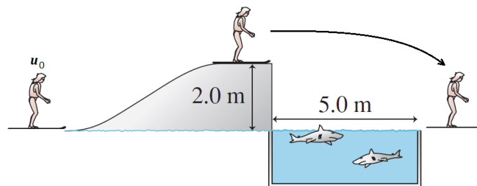
Σχήμα 2.68: Ακροβατικό άλμα.
