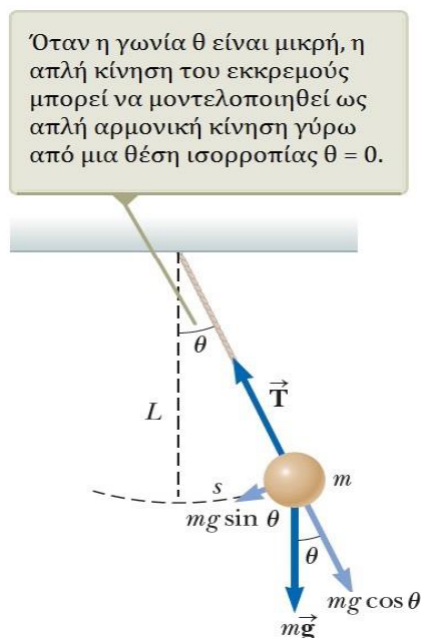
Σχήμα 3.16: Εκκρεμές.
