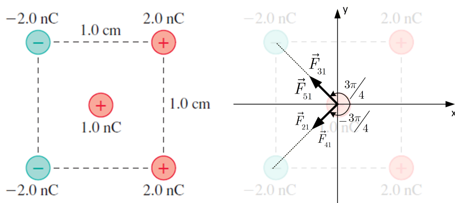
Σχήμα 4.91: Πεντάδα φορτίων.
