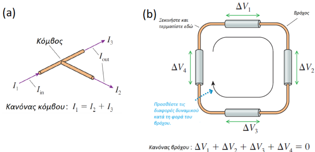
Σχήμα 4.74: (a) 1ος Κανόνας Kirchhoff - κανόνας κόμβου, (b) 2ος Κανόνας Kirchhoff - κανόνας βρόχου).
