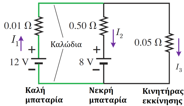
Σχήμα 4.83: Κύκλωμα με ρεύματα Άσκησης 4.45.
