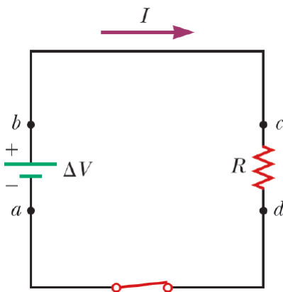
Σχήμα 4.69: Απλό κύκλωμα μπαταρίας - αντιστάτη.
