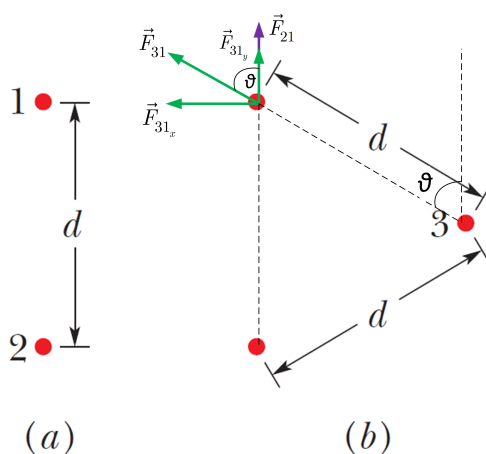
Σχήμα 4.95: Σχήμα Λύσης Άσκησης 4.57.
