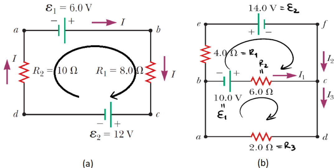
Σχήμα 4.76: (α) Κύκλωμα και δυο αντιστάτες, (β) κύκλωμα με τρεις αντιστάτες.
