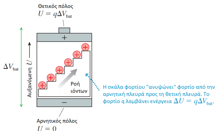
Σχήμα 4.68: Μοντέλο μπαταρίας - σκάλας.
