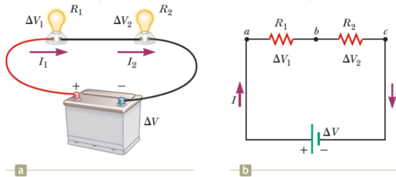
Σχήμα 4.64: Συμβολισμός αντιστάτων σε κύκλωμα.
