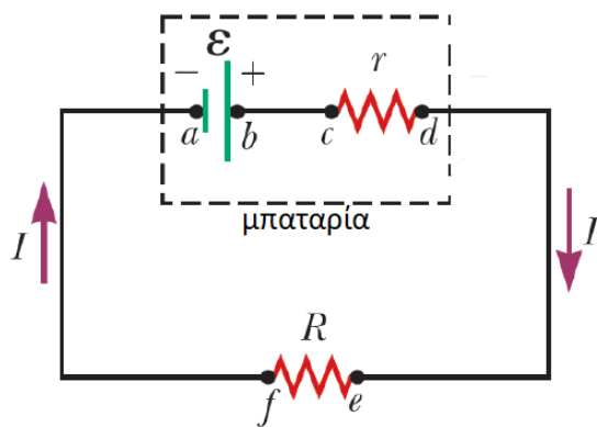
Σχήμα 4.72: Μοντέλο μπαταρίας σε κύκλωμα με αντιστάτη.
