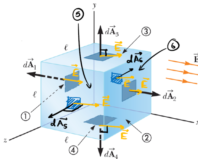
Σχήμα 4.24: Κύβος σε ηλεκτρικό πεδίο.
