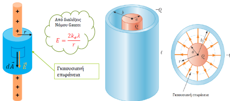
Σχήμα 4.54: Κυλινδρικός πυκνωτής.
