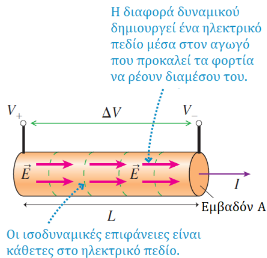
Σχήμα 4.63: Ρεύμα και διαφορά δυναμικού.
