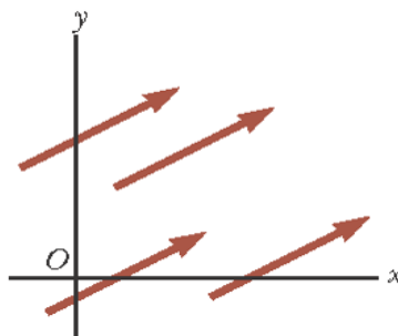
Σχήμα 1.2: Ίσα διανύσματα.
