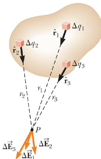
Σχήμα 4.10: Κατανομή φορτίου.
