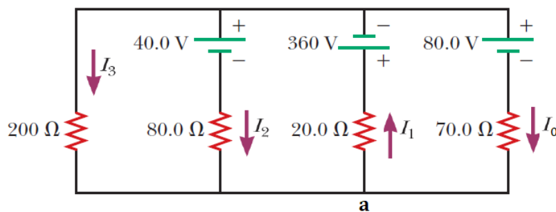
Σχήμα 4.78: Κύκλωμα και κανόνες Kirchhoff.
