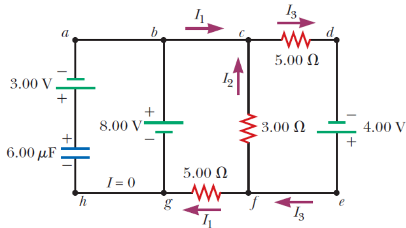
Σχήμα 4.87: Κύκλωμα αντιστάσεων και πυκνωτών.
