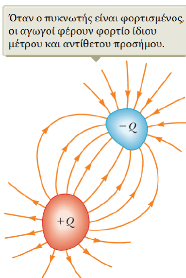
Σχήμα 4.50: Φορτισμένοι αγωγοί σε διάταξη πυκνωτή.
